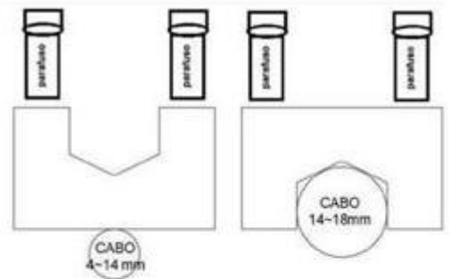
FORMA DE FIXAÇÃO DA PRESILHA NO CABO DE AÇO
